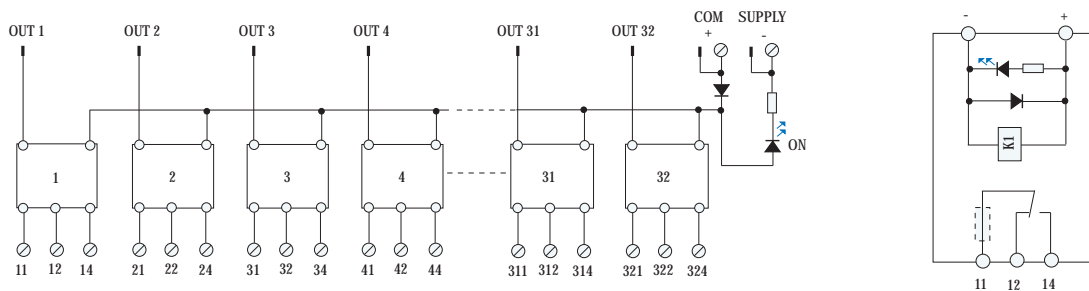
SCHEMA A BLOCCHI MODULI 32 USCITE 32 OUTPUT MODULES BLOCK DIAGRAMS
